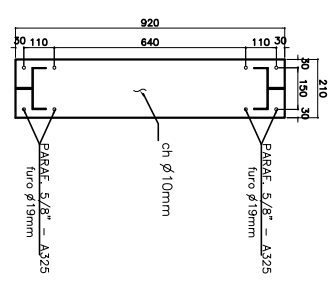
Det. Ligação entre Tesouras
