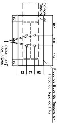
Ligação Tesoura-Pilar
